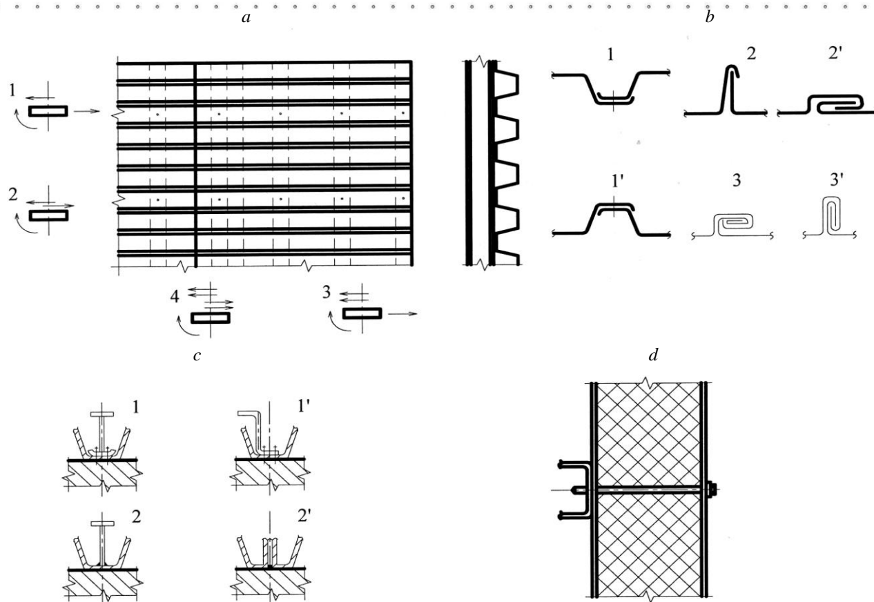
a - фрагмент конструкции покрытия со стальным профилированным настилом и схема действия сил на опорах (1- соединения в среднем участке; 2 и 3- соединения соответственно по продольным и поперечным полкам; 4 - соединения в месте пересечения продольных и поперечных полок); b - схема соединений по продольным полкам (1 и 1 1 - при расположении полок внахлест в нижнем и верхнем положениях соответственно для утепленных и холодных покрытий; 2 и 2 1 - простой стоячий и лежащий фальцы; 3 и 3 1 - двойной фальц, стоячий и лежащий); c - сдвигоустойчивые элементы (1 и 1 1 - на высокопрочных дюбелях; 2-на контактной сварке; 2 1 - на дуговой сварке); d - фрагмент трехслойной стеновой панели на самосверлящем винте
